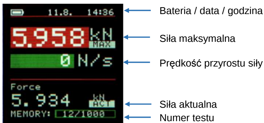
Ekran cyfrowy
