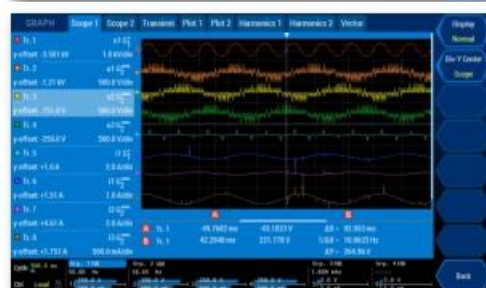
Wyświetlanie wartości próbkowania 16 sygnałów w Scope 1 i Scope 2
