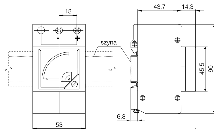
Rys. 1. Wymiary zewnętrzne mierników MB16
