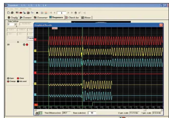
Instrument wizualizacji zaburzeń (Transient)
