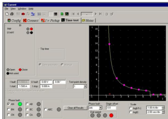
Instrument prądowy – pomiar czasu działania
