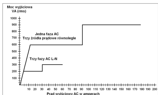
Charakterystyka mocy źródeł prądowych FREJA 543
