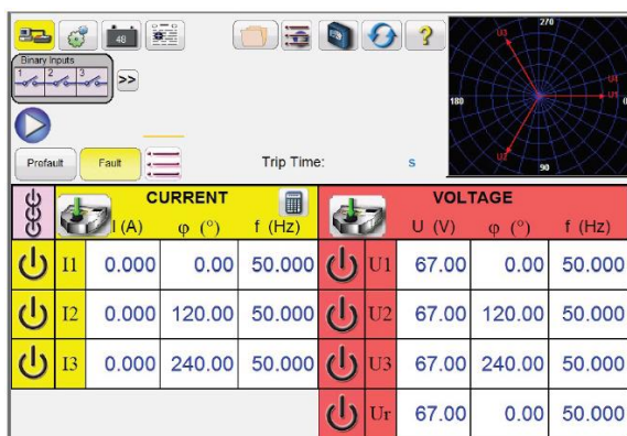
Interfejs użytkownika w aplikacji FREJA Local
