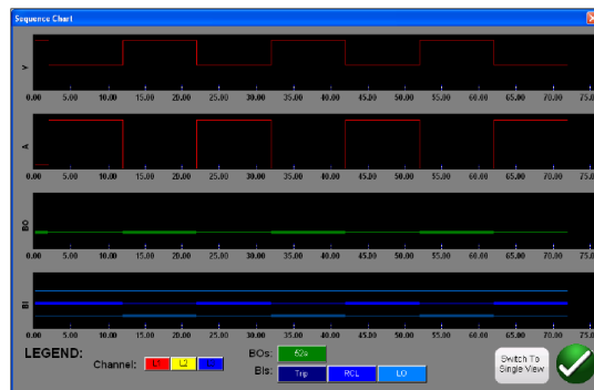
Przykładowy obraz zaprogramowanej sekwencji napięć, prądów oraz stanów na wejściach i wyjściach binarnych
