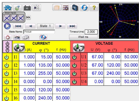
Ekran testów sekwencyjnych
