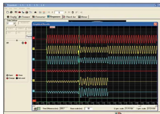
Instrument wizualizacji zakłóceń (Transient)
