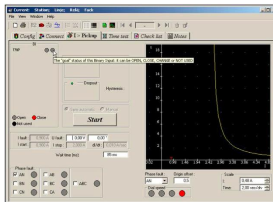
Instrument prądowy – pomiar prądu rozruchowego
