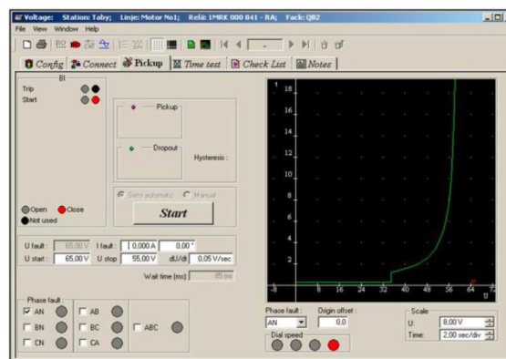
Instrument napięciowy – pomiar napięcia pobudzenia
