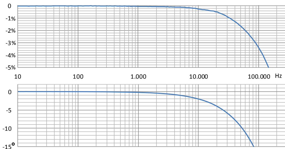
Gain/Phase
