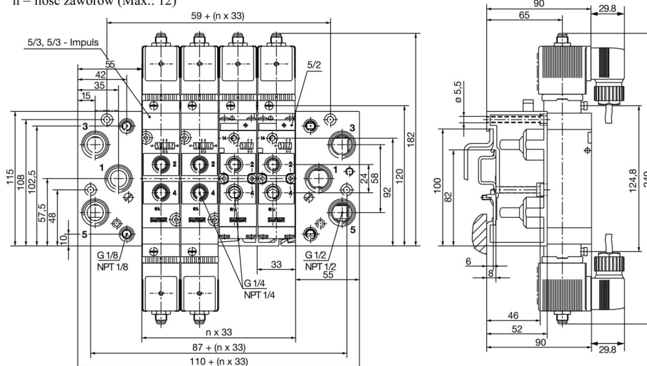
Wymiary bloku zaworowego i montaż naścienny (rozstaw zaworów: 33 mm) [mm]:
