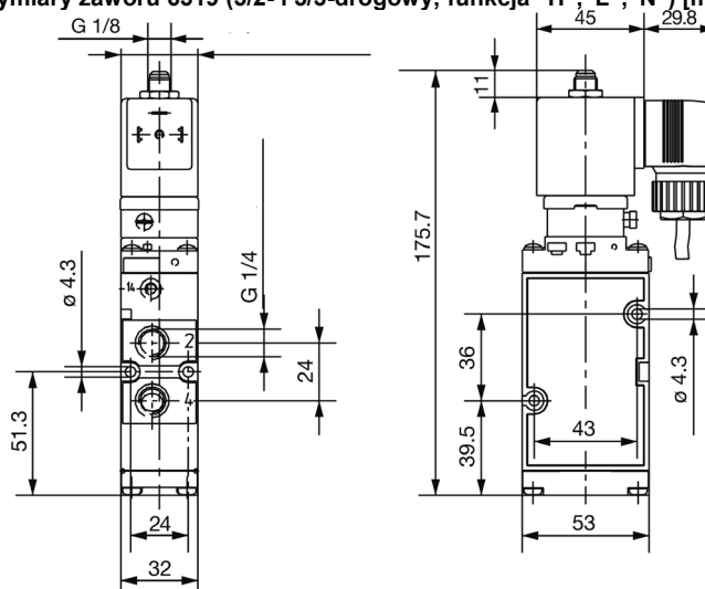
Wymiary zaworu 6519 (5/2- i 5/3-drogowy; funkcja "H","L","N") [mm]:
